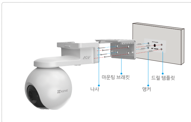
그림 2 벽 장착
