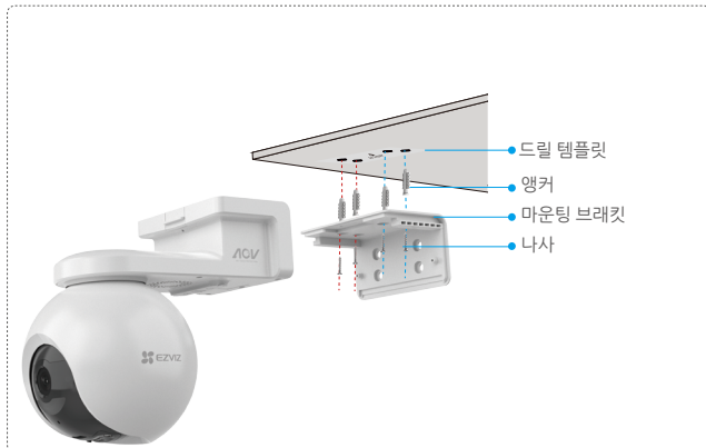
그림 1 천장 장착
